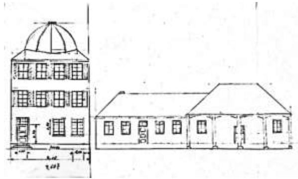
Aufriss Prinzessinnenpalais mit Wache Innenhof
